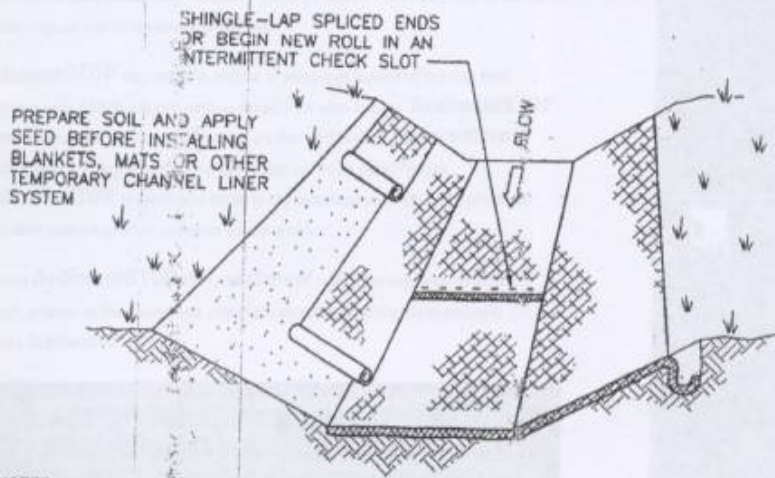
LONGITUDINAL ANCHOR TRENCH
